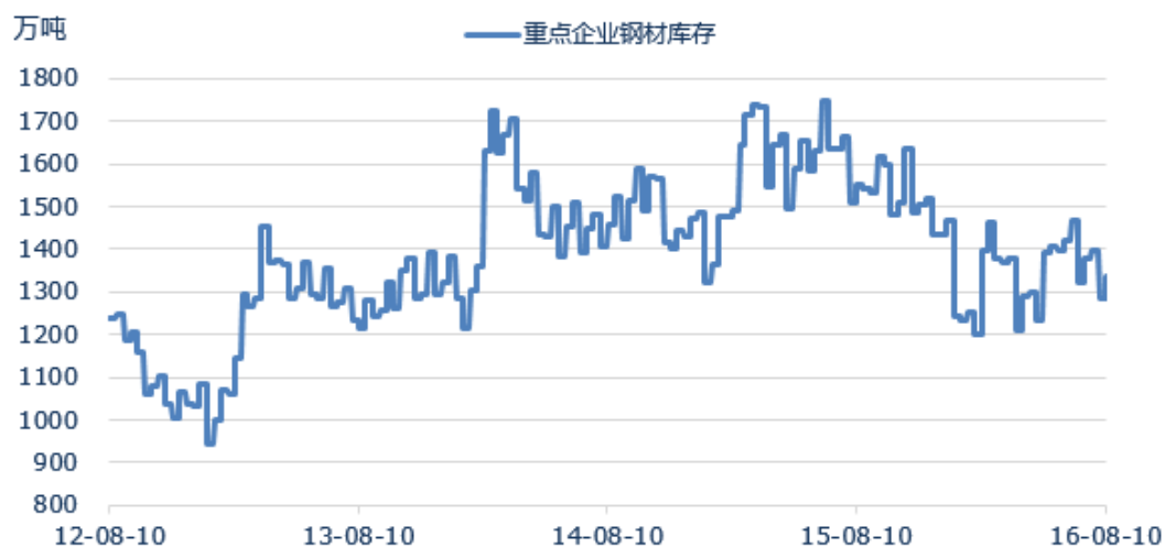
图5：重点企业钢材库存相对偏低
